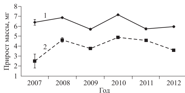
Рис. 3. Динамика прироста фитомассы мха H. splendens (1 – под кронами; 2 – в межкроновом пространстве).
